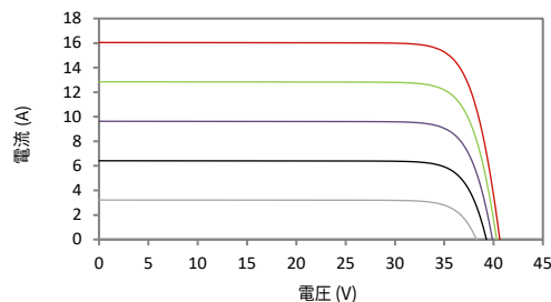
電流-電圧曲線 (54QL6-DV 535 W)
