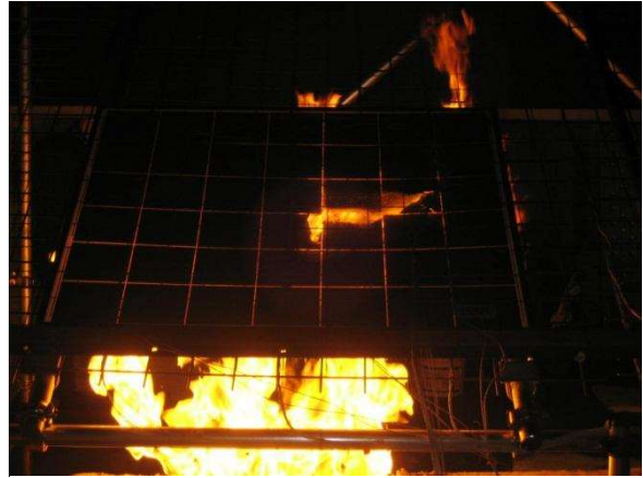
写真5-8 Test-5_A1 加熱4分時の状況
