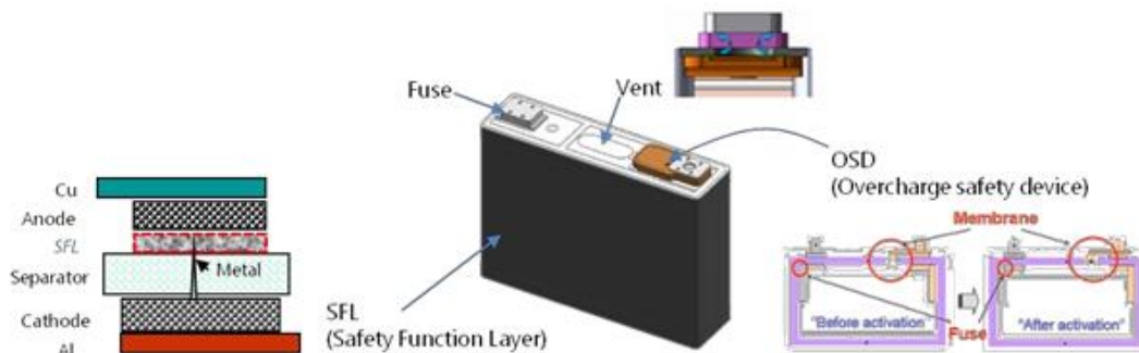
図 4-7 安全設計
