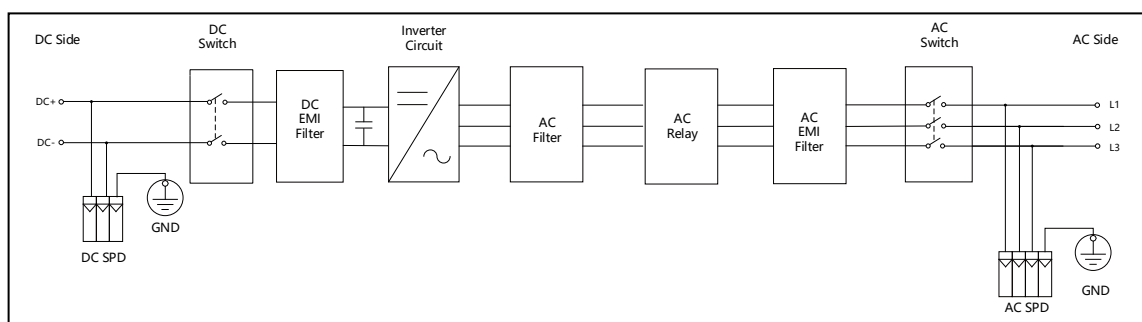
図 3-2 SC50HV 主回路
