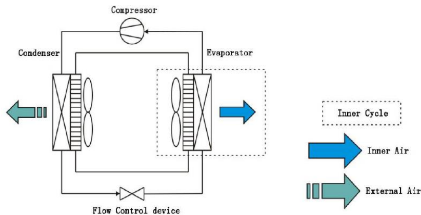
図 6-1 HVAC 動作原理図
