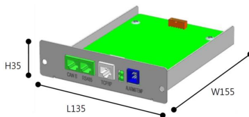
図 4-6 システム BMS
